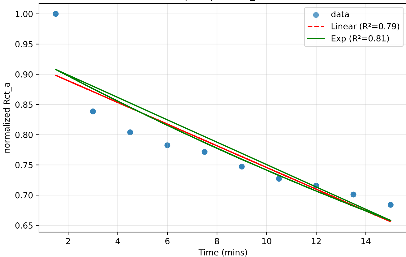
Chip 39 | 100nM_asso
